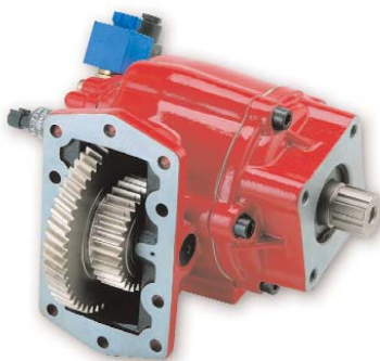
מעבירי כוח SLICK-SHIFT לתמסורות ALLISON סדרת MD
