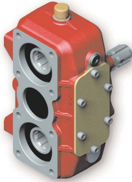
יחידת פיצול ל-2 משאבות דגם ISO
